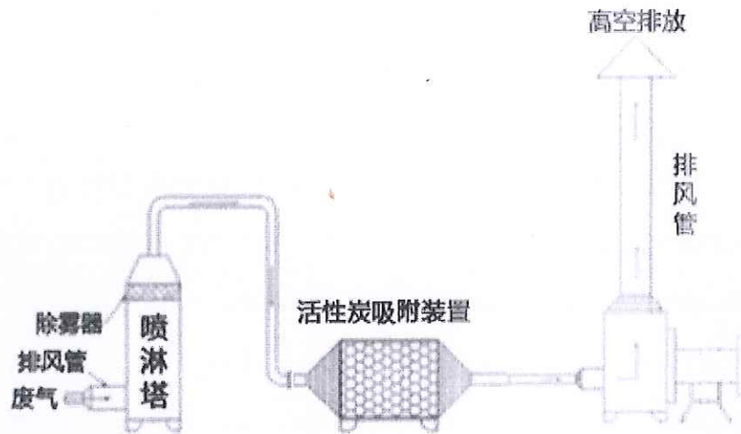
有机废气废气处理工艺流程
