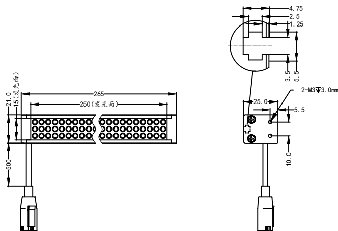
螺母槽尺寸图
