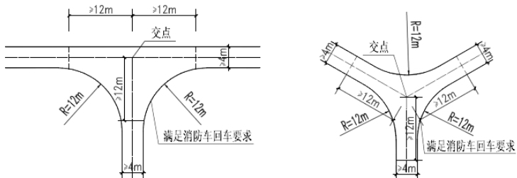
附图 1 不规则的消防回车场地
